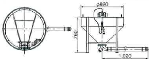
■外形寸法図
