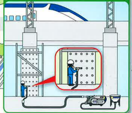
耐震補強工事
