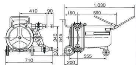
■外形寸法図
