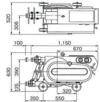
■外形寸法図
