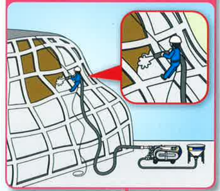
法面吹付
