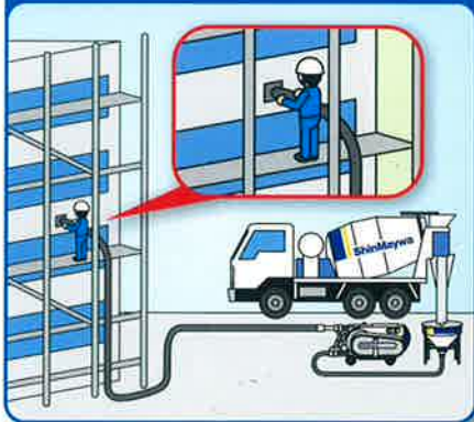
モルタル搬送
