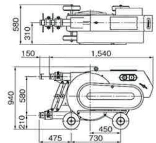
■外形寸法図
